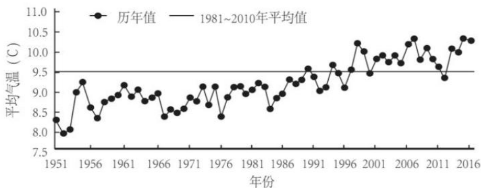
1951~2016年全国年平均气温年际变化
